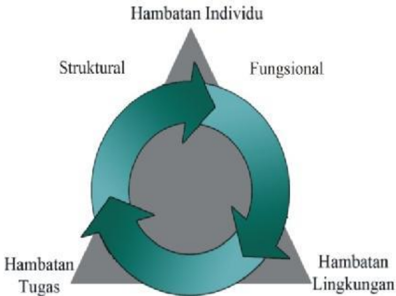
Gambar 12.3. Model Segitiga Faktor Interaksi yang Mempengaruhi Gerak
