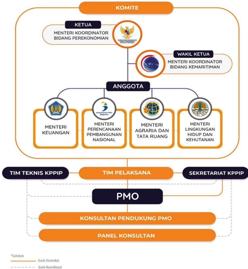
Gambar 14.1: Struktur KPPIP
